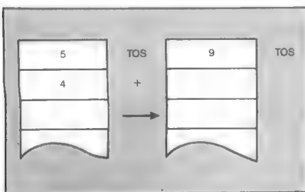
Bild 1. So verändert sich der Stack bei der Addition
